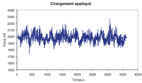
Contrôle direct de vérin hydraulique pour simuler le chargement en mer
