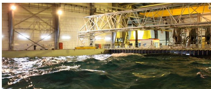
Bassin de Houle et de Génie Océanique © Centrale Nantes
